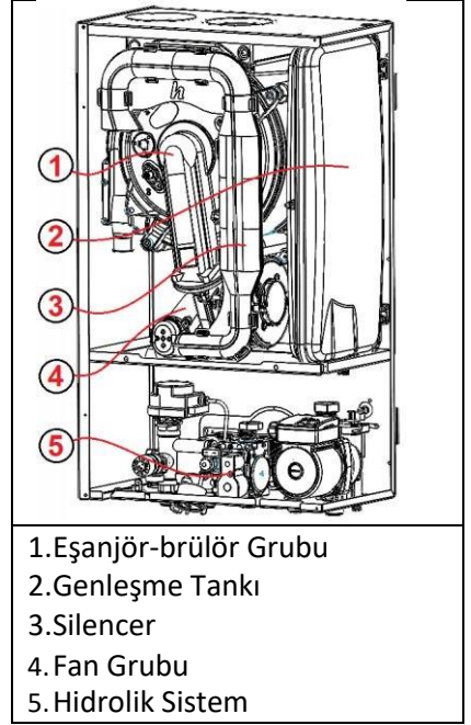
Şekil 1.4.2: Cihaz Tanımı
