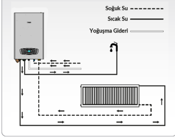
Şekil 5.2 Bağlantılar
