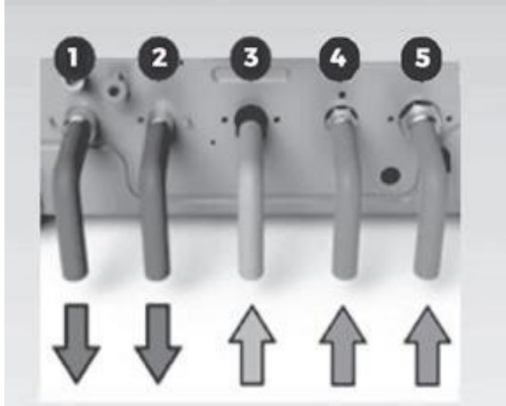
Şekil 5.2 Bağlantılar
